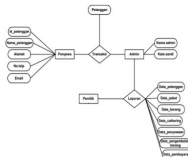
Gambar 4. ERD Diagram Sistem Penyewaan
